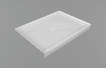
BG-NEPSB-3648 3F SIZE: 1213x911x103mm
