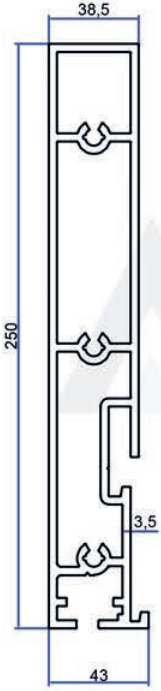
Cod: 2088 - 7,213 kg/m 250'lik Oluk Dikmesi 250' Groove Sewing
