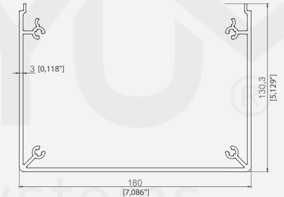
DİKME GÖVDE PROFİLİ / PILLAR MAIN PROFILE
