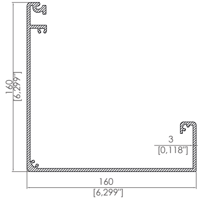
Motor Kutusu Motor Box
