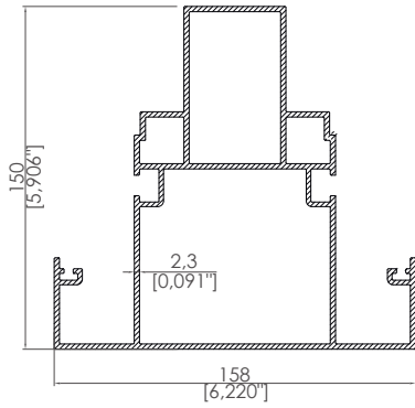
Orta Taşıyıcı Profili Middle Beam Profile
