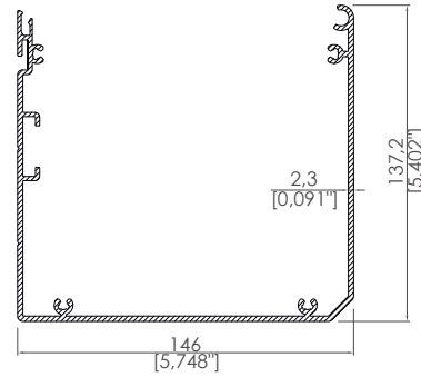
Motor Kutusu Motor Box
