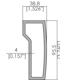
38,8x95,5 Dere Eki Profili 38,8x95,5 Gutter Profile Connection
