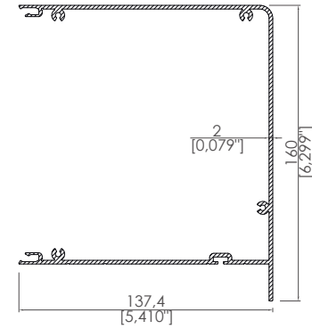
Motor Kutusu Profili Motor Box Profile
