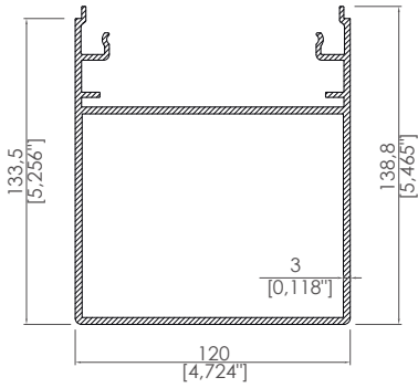
Yan Kayıt Profili Side Beam Profile
