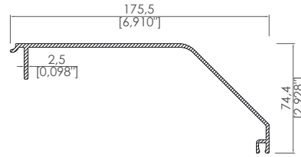
Motor Kutusu Kapağı Motor Box Cover
