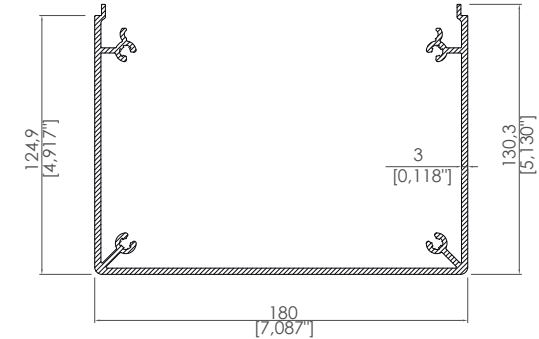
Dikme Gövde Profili Pillar Main Profile
