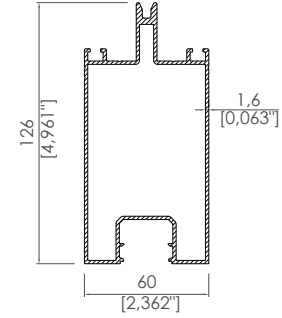
Şerit Ledli Cam Taşıyıcı Profili Glass Carrier Profile Linear Led
