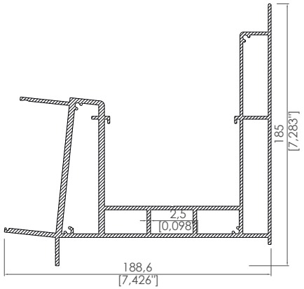
188x185 Düz Dere 188x185 Gutter Profiler
