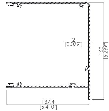
Motor Kutusu Profili Motor Box Profile
