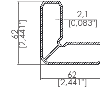
Kasa Köşe Takoğu Profili Frame Corner Block Profile
