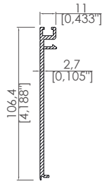
11x106,4 Dere ve Arka Kayıt Kapağı 11x106,4 Gutter and Back Beam Cover Profile
