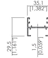
Orta Panel Birleştirme Profili Middle Panel Connection Profile
