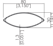
80x30 Güneş Kırıcı Profili 80x30 Sun Breaker Profile
