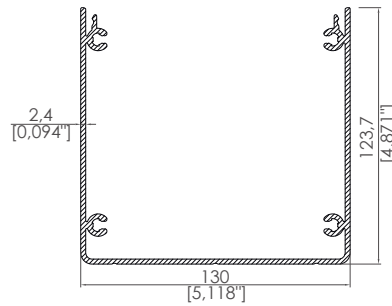
120x123 Dikme Gövde 120x123 Pillar Main
