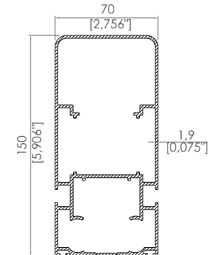
70x150 Eko Ray 70x150 Eco Rail Profile
