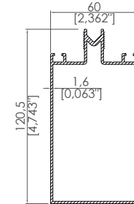
Standart Cam Taşıyıcı Standart Glass Carrier Profile
