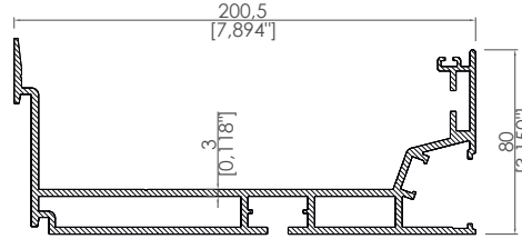
Dere Profil Gutter Profile
