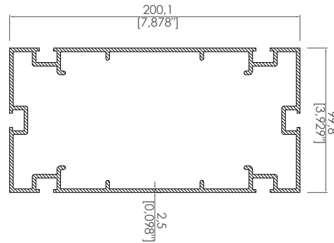
Arka Kayıt Back Beam
