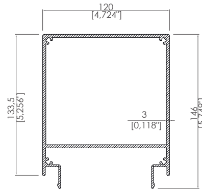
Yan Kayıt Üst Profili Side Beam Top Profile
