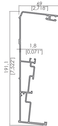
69x191 Arka Kayıt 69x191 Back Beam
