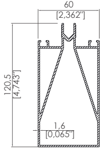
Destekli Cam Taşıyıcı 1 Supported Glass Carrier Profile 1
