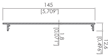
Motor Kutusu Kapak Profili Motor Box Cover Profile
