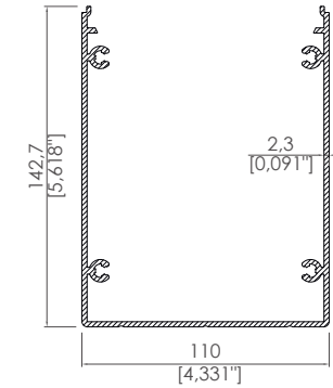
110x145 Dikme Gövde 110x145 Pillar Main Profile
