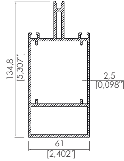
61x134,8 Cam Taşıyıcı 61x134,8 Glass Carrier Profile
