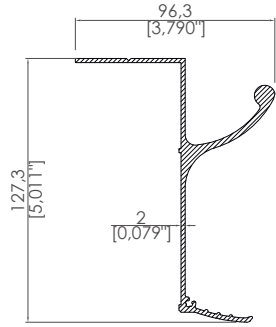
Arka Kayıt Bağlantı Ray Profili Rail - Back Beam Connection Profile
