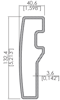
40,6X132,4 Dere Eki Profili 40,6X132,4 Gutter Profile Connection
