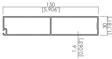
30x150 Kutu Profil 30x150 Box Profile
