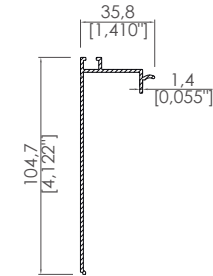
35,8x104,7 Dere ve Arka Kayıt Kapağı 35,8x104,7 Gutter and Back Beam Cover Profile
