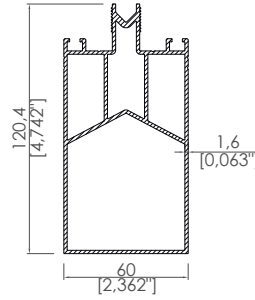
Destekli Cam Taşıyıcı 2 Supported Glass Carrier Profile 2
