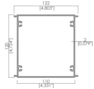
122x120 Dikme Gövde Profili 122x120 Pillar Main Profile
