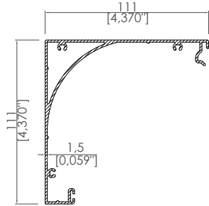
Motor Kutusu Profili Motor Box Profile
