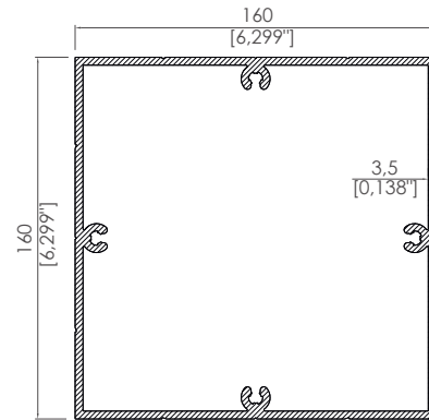
Çizgili Dikme Profili Lined Pillar Profile
