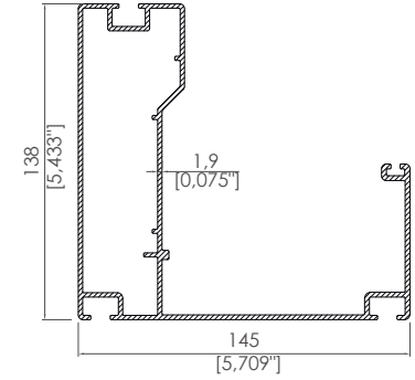
138x145 Eko Dere 138X145 Eco Gutter
