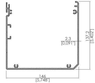
Motor Kutusu Motor Box
