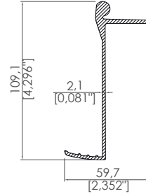
Dere Bağlantı Ray Profili Rail - Gutter Connection Profile
