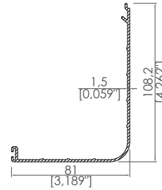
Motor Kutusu Kapağı Profili Motor Box Cover Profile
