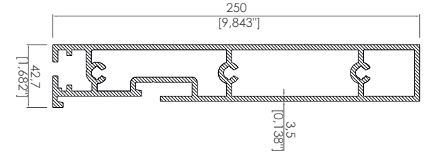
Yan Kayıt Profili Side Beam Profile
