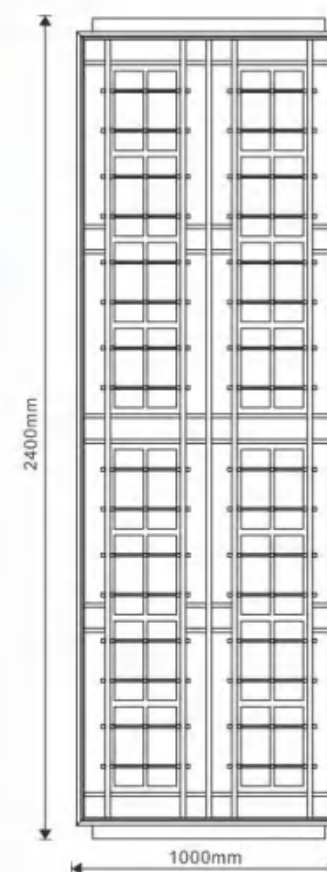
Product No.: YA 007 Standard size: W1000*H2400*D70mm 材质: 304不锈钢 建议颜色: 拉丝玫瑰金/拉丝香槟金/拉丝枪黑
