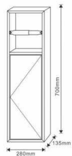
Product No.: BK 003 Standard size: W280*H700*D135mm 材质: 304不锈钢 建议颜色: 拉丝玫瑰金/拉丝香槟金/拉丝银钛
