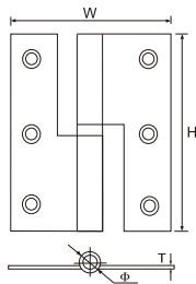
SB-L2 铜直角(L)铰
