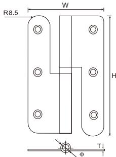
SB-L3 铜圆角(L)铰
