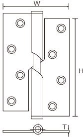
SS-RH Rising Hinge 自升铰链
