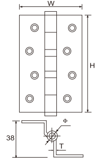
SB-CK3 铜曲铰
