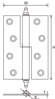
SB-L4 铜直角(L)铰
