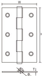
SB426 铜家居铰链
