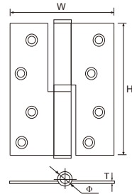
SB-L5 铜直角(L)铰
