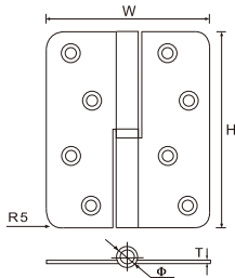
SB-L1 铜圆角(L)铰
