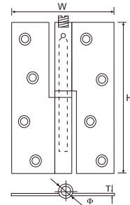
SB-L6 铜可调节直角(L)铰
