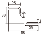
SS-CK1 不锈钢曲铰链
