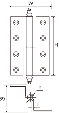
SB-CK2 铜曲铰
