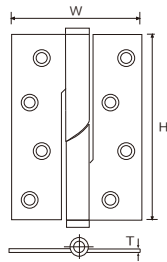
SS-FH Falling Hinge 自降铰链
